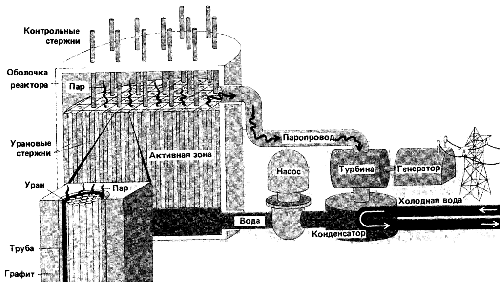
Принципиальная схема реактора РБМК
